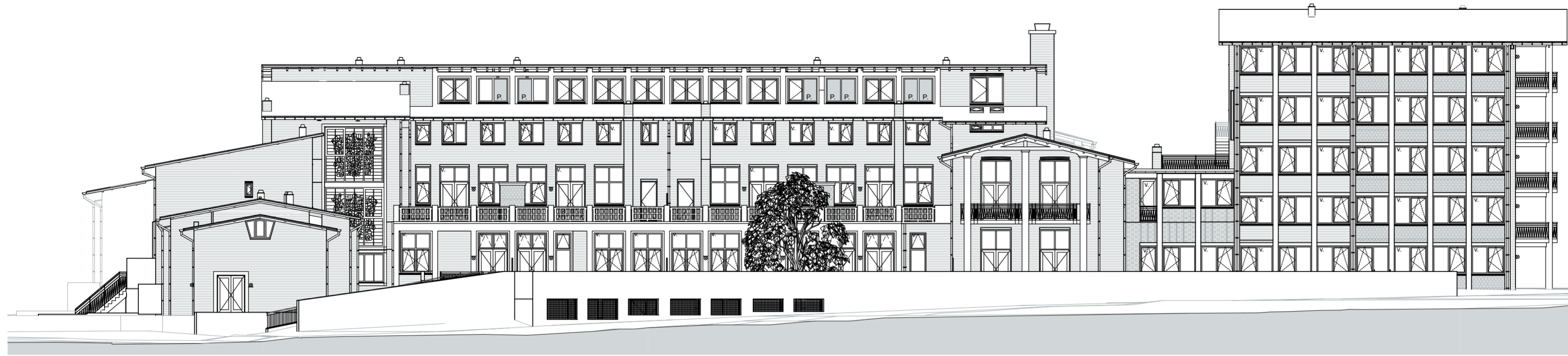
OOSTGEVEL
