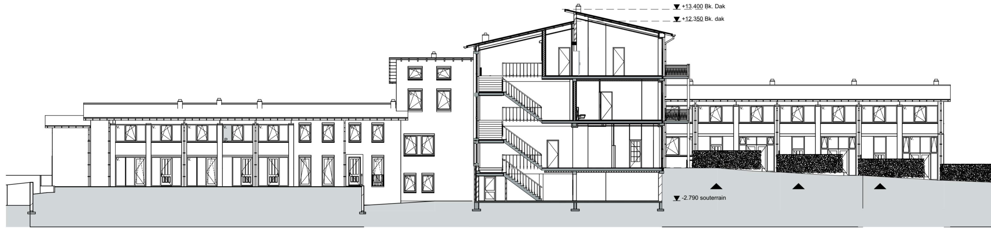
DOORSNEDE I-I NOORDGEVEL BOUWDELEN 01 & 03
