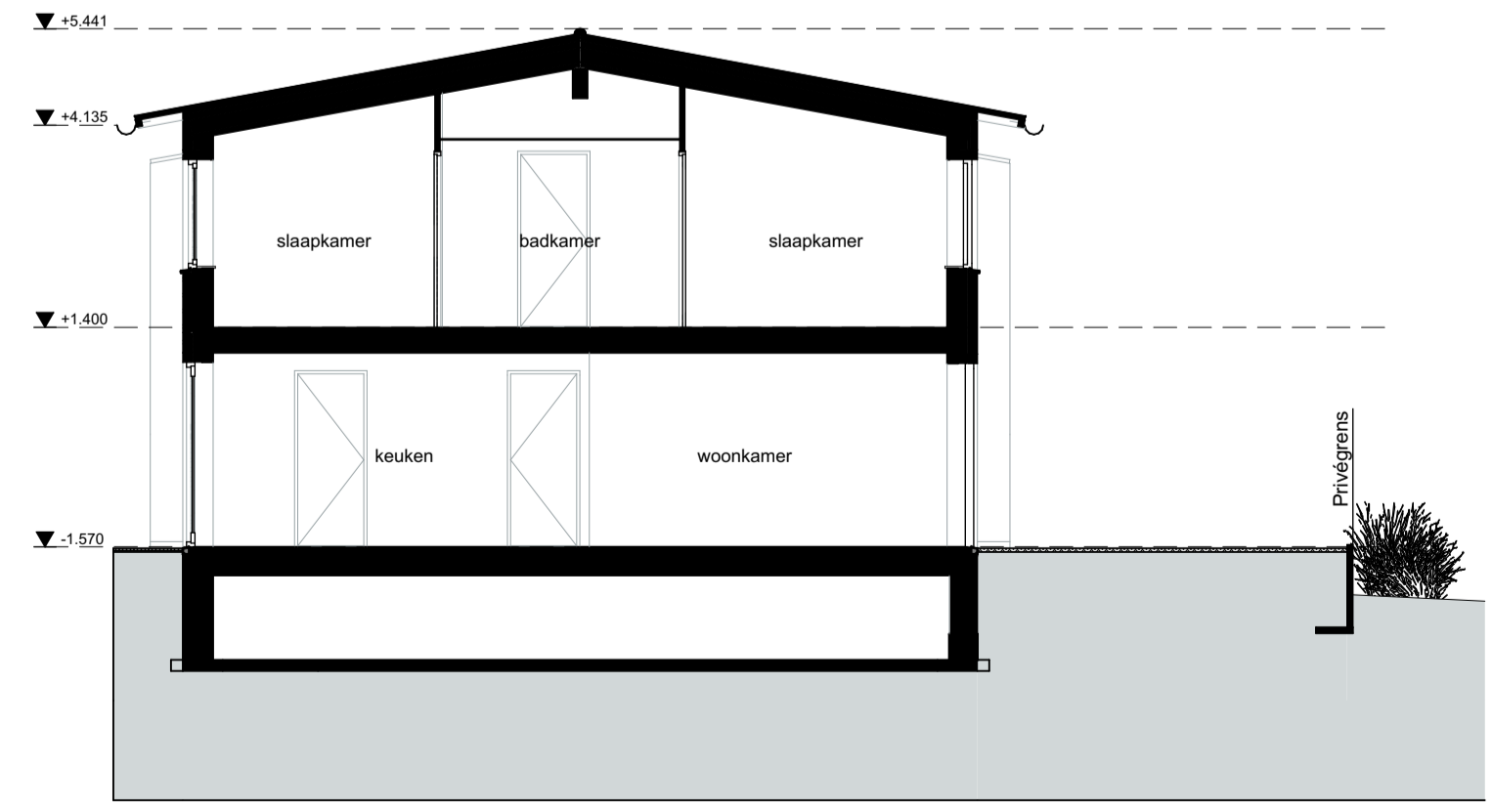
Doorsnede J103
